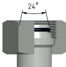
Dichtkegelanschlüsse DKOL/DKOS 24° mit O-Ring und Überwurfmutter Conical seal connection DKOL/DKOS 24° with O-ring and union nut
